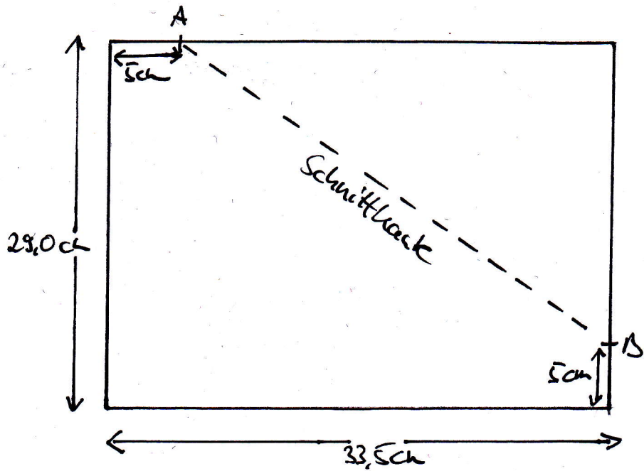
Schemazeichnung 1
